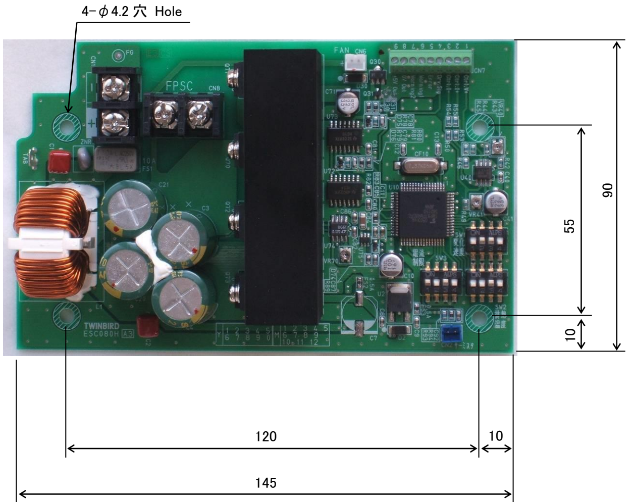
(b) 駆動基板 Drive PCB
