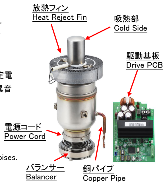
SC-TD08 スターリングクーラー 08 SC-TD08 Stirling Cooler 08
